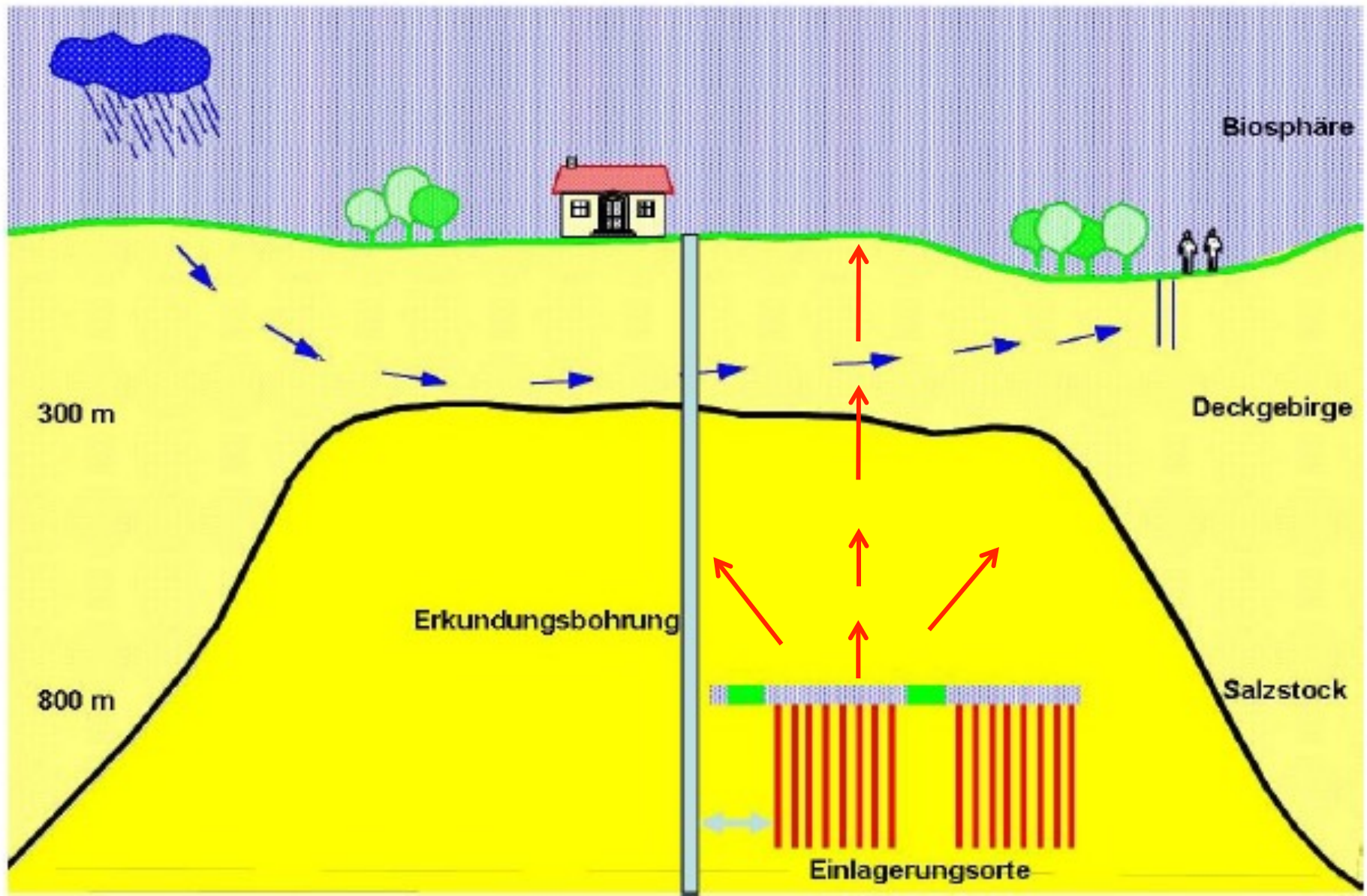
Schemat. Schnitt durch das Endlager mit Wirts- u. Deckgestein (GRS 2008)
